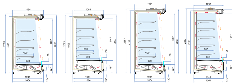
Palco P105/H205 F30 L125-188-220-250-375
